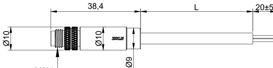
公针头
