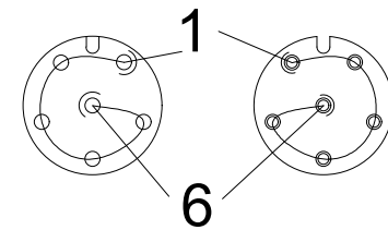
孔母头
